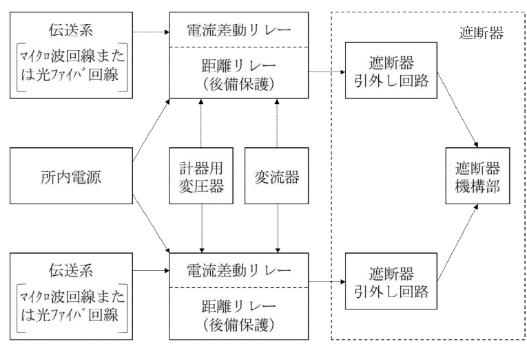
第三-9図 送電線保護リレー装置の2系列化(例)
