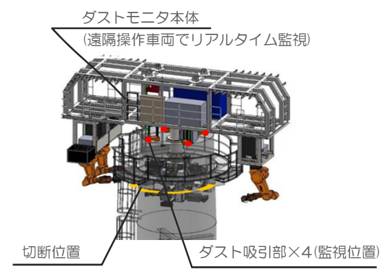
A部分(筒身解体ツール)拡大
