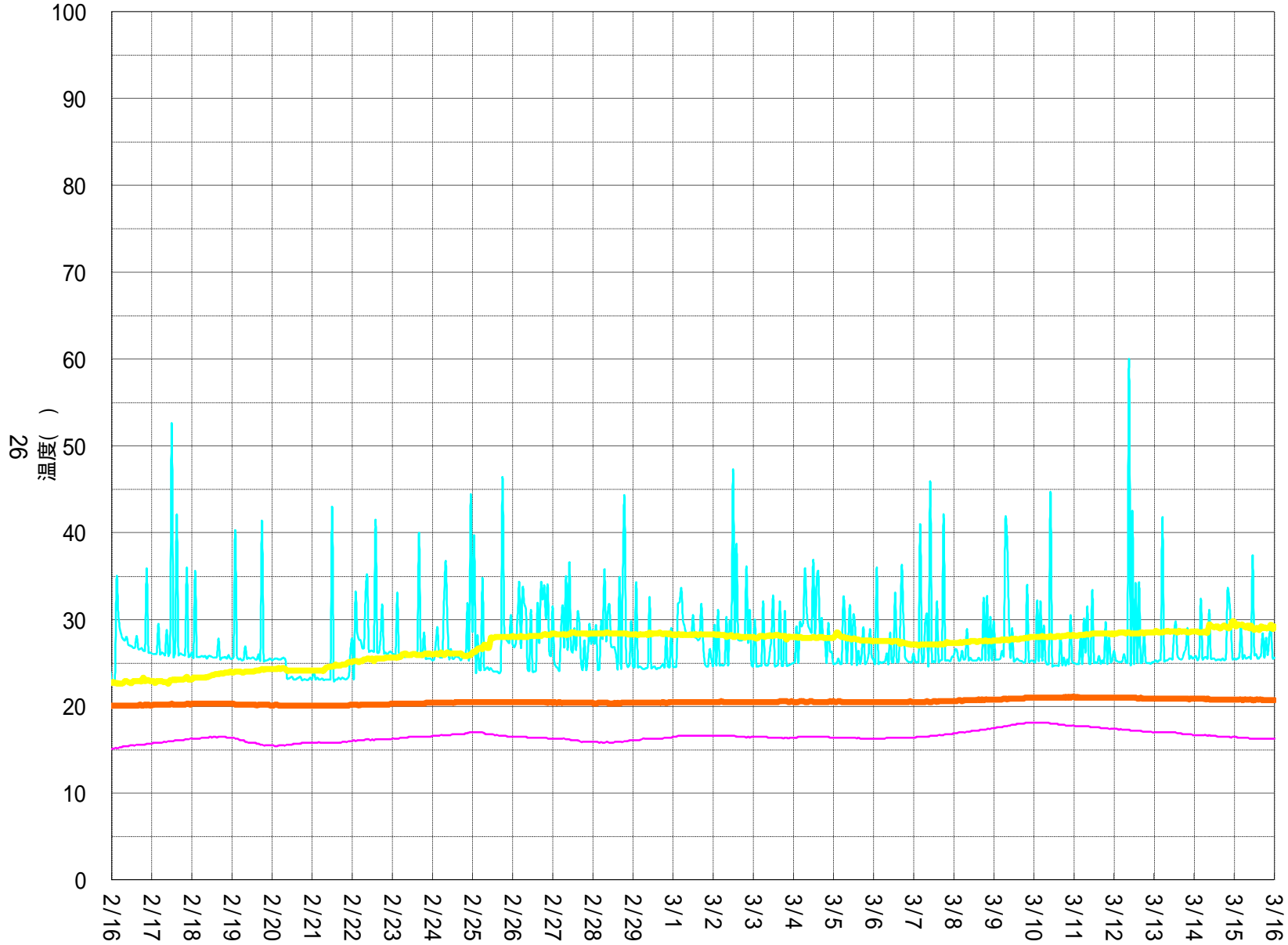
2号機 RPV周辺温度計(下部)
