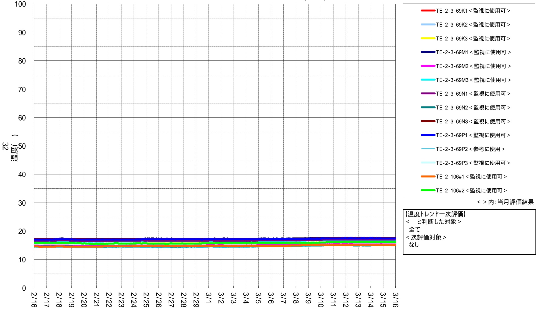
3号機 RPV周辺温度計(下部)
