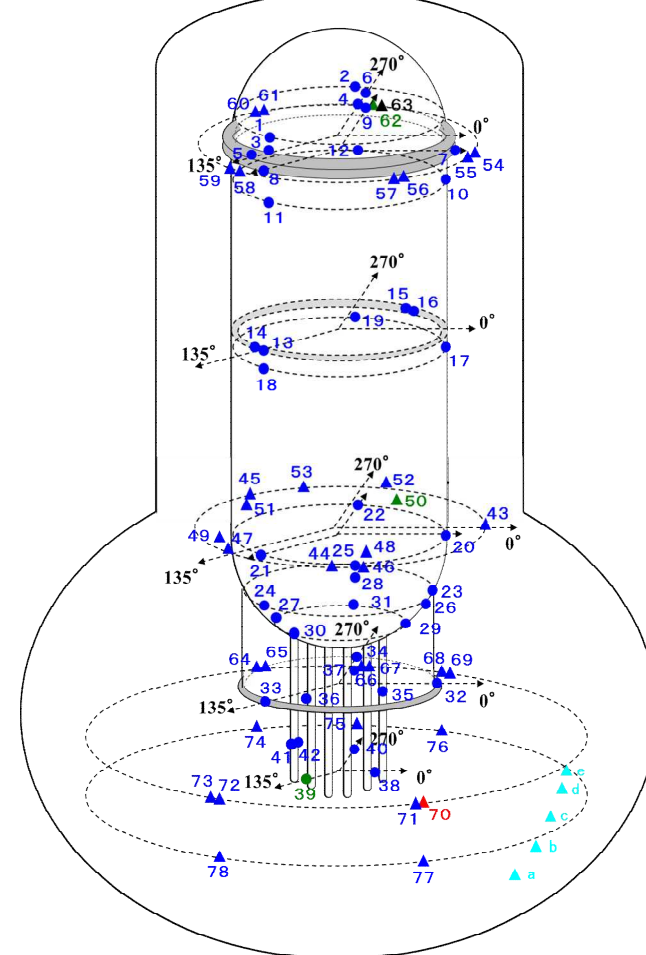
<立体図>
