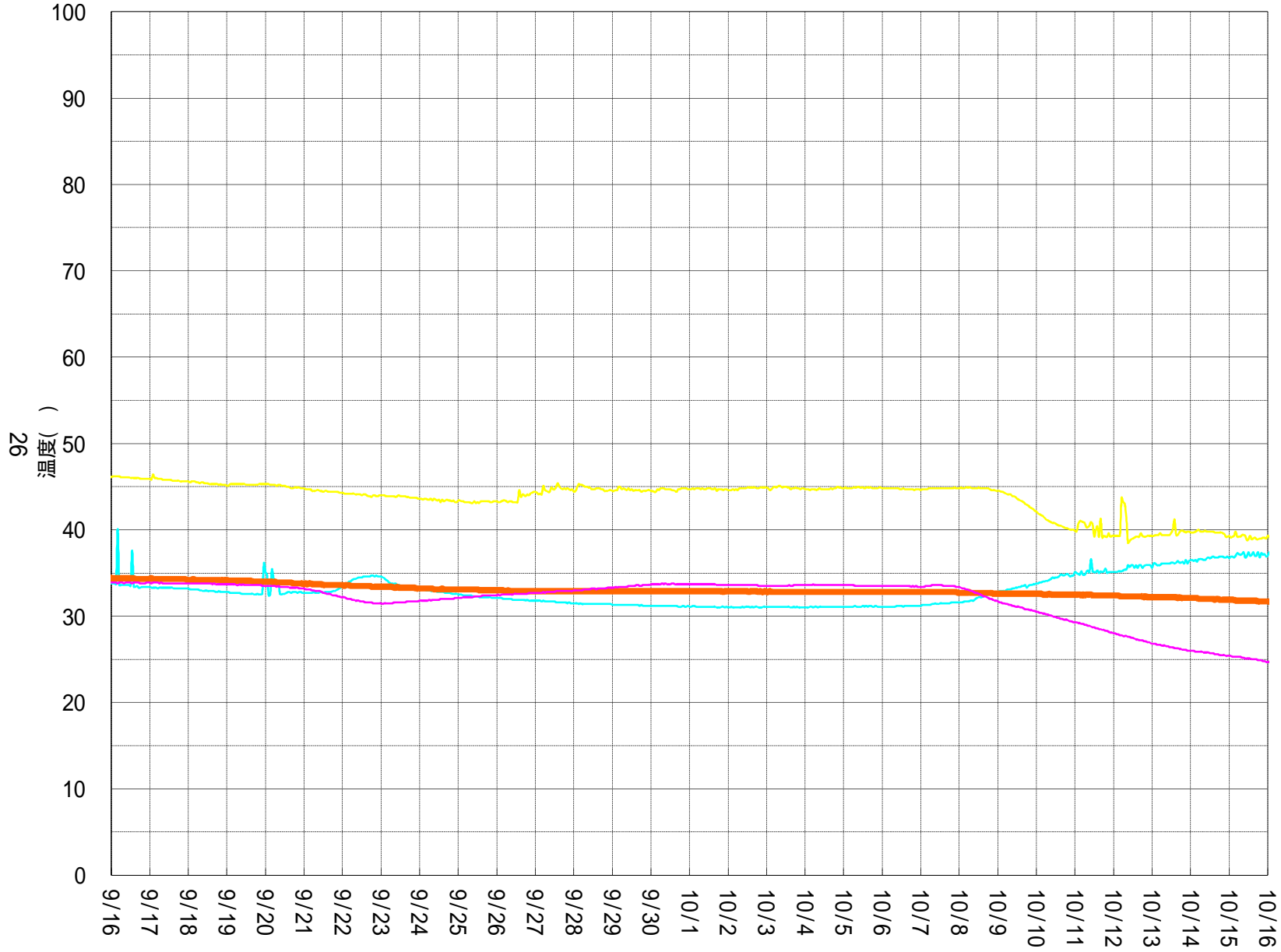
2号機 RPV周辺温度計(下部)
