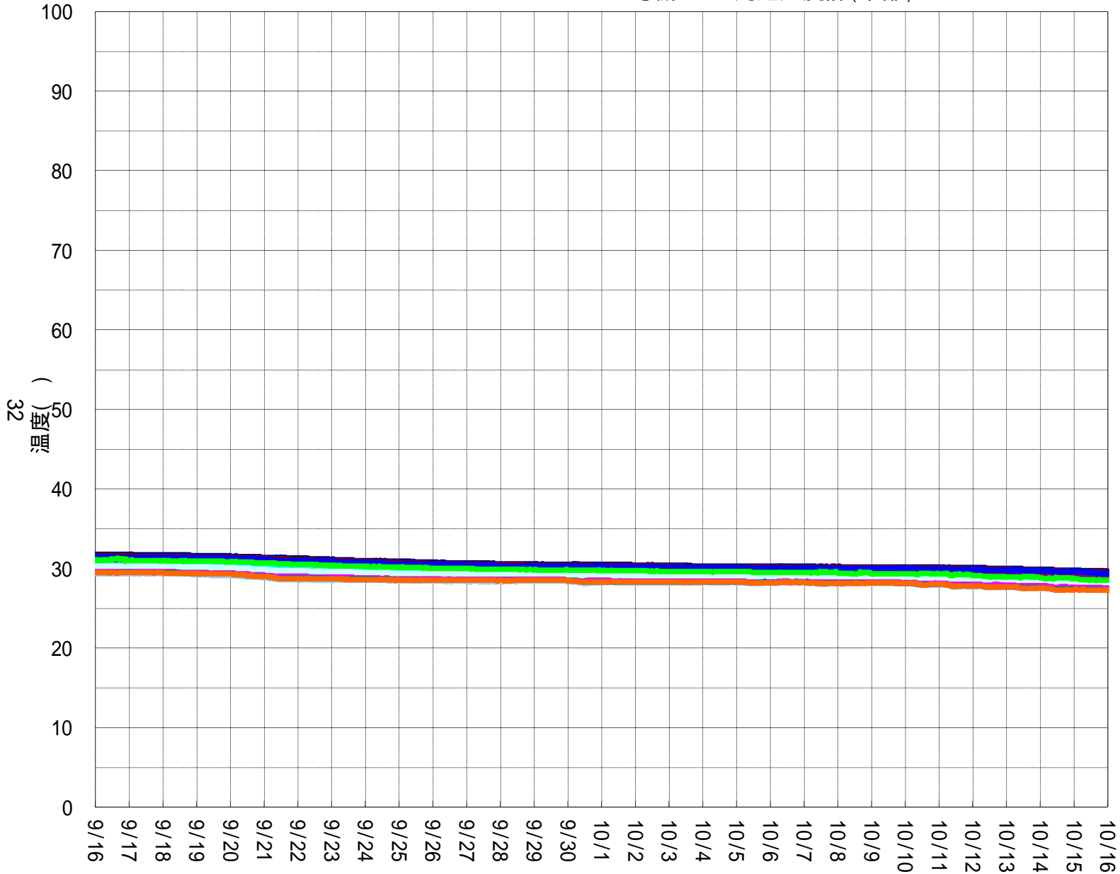
3号機 RPV周辺温度計(下部)
