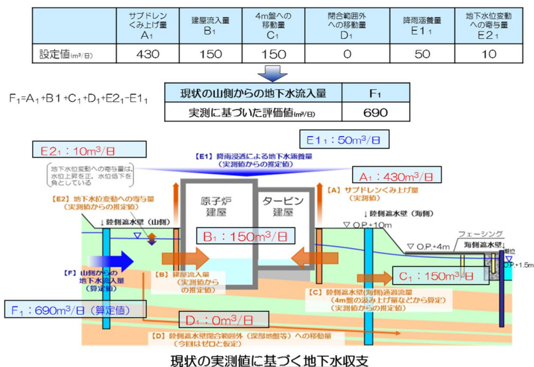
図－2 一部閉合（Ⅱ）実施前の山側からの地下水流入量の想定
