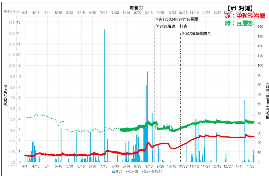
図一八． 6 中粒砂岩層／互層部，細粒・粗粒砂岩の水頭比較（海側①）
