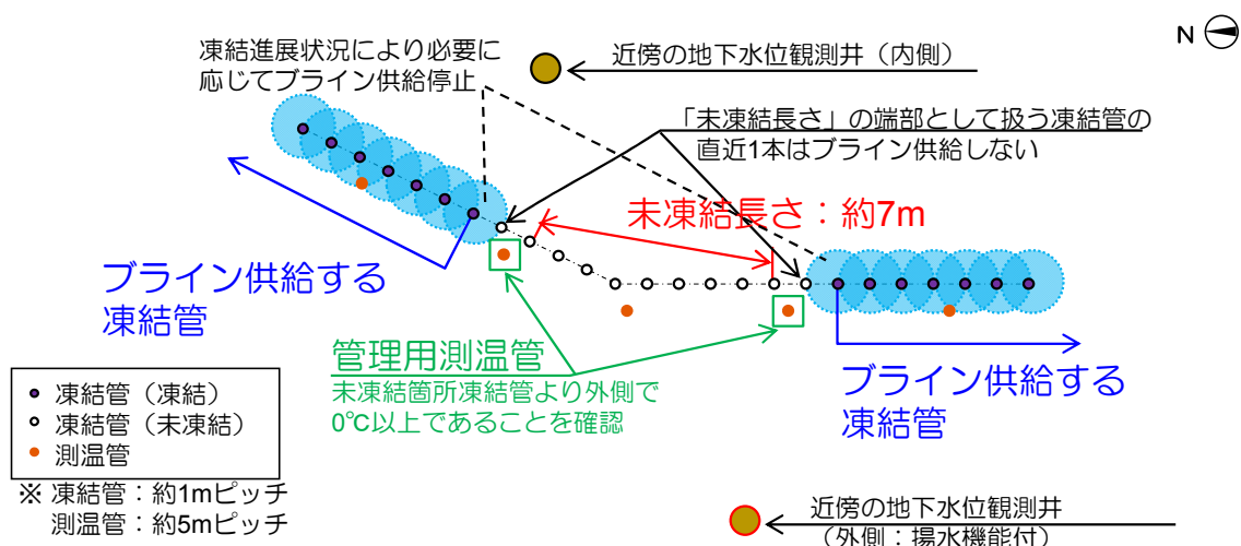
図－ 1 7 未凍結長さの管理図（例：西側③）
