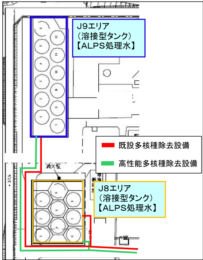
タンクエリア詳細図
