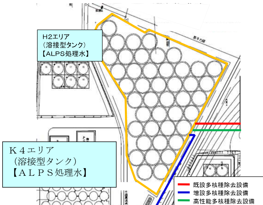
タンクエリア詳細図
