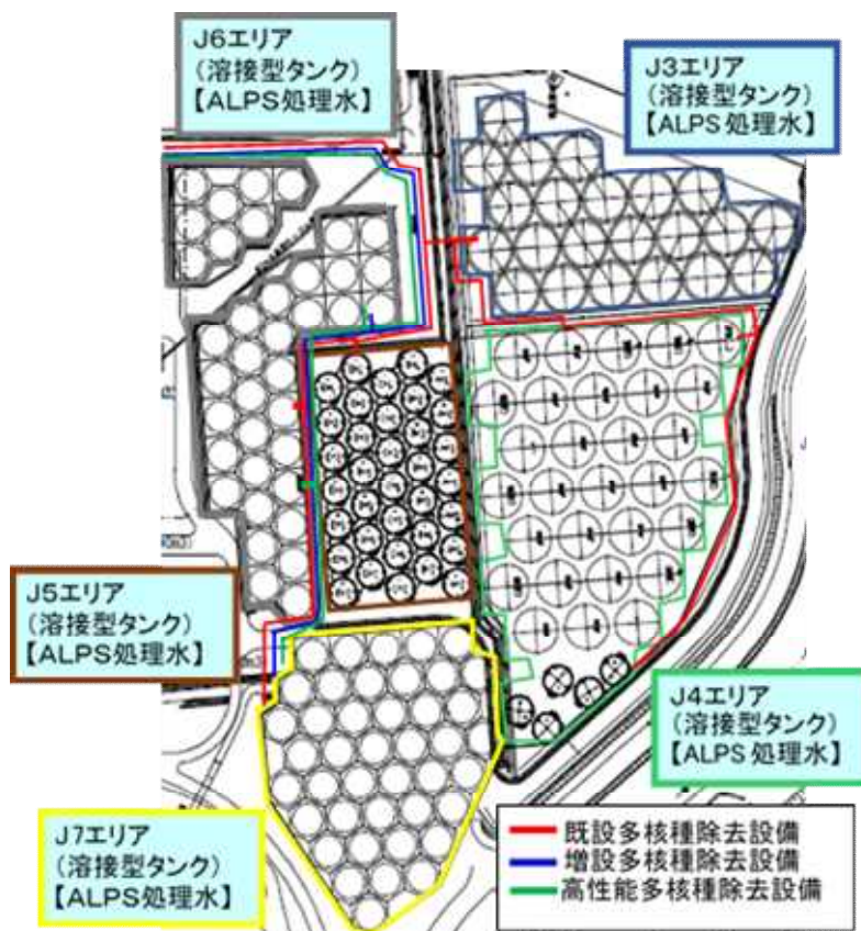
タンクエリア詳細図
