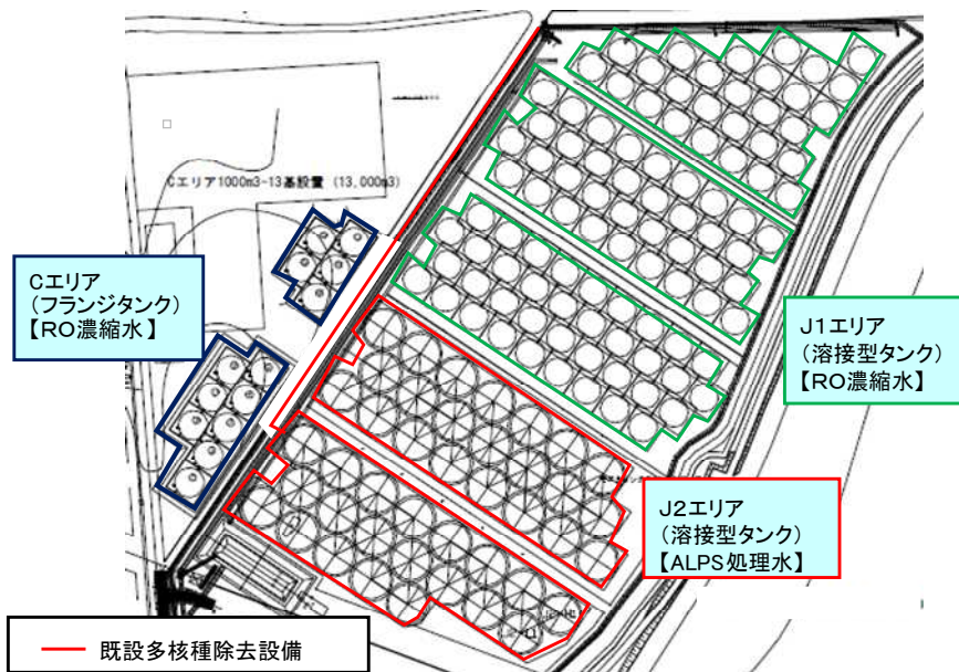
タンクエリア詳細図
