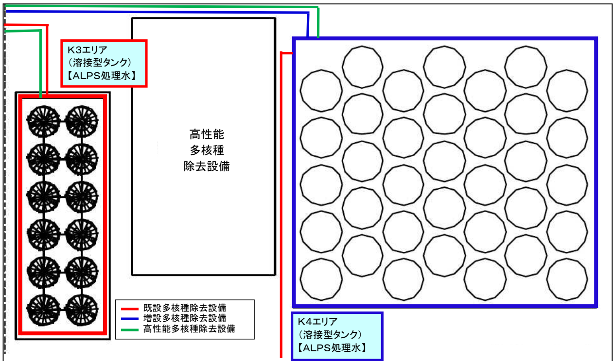
タンクエリア詳細図
