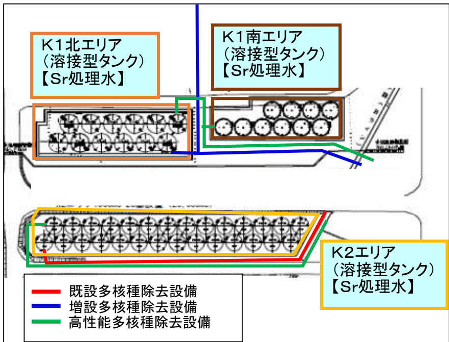
タンクエリア詳細図
