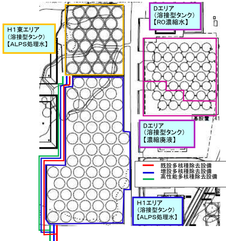
タンクエリア詳細図
