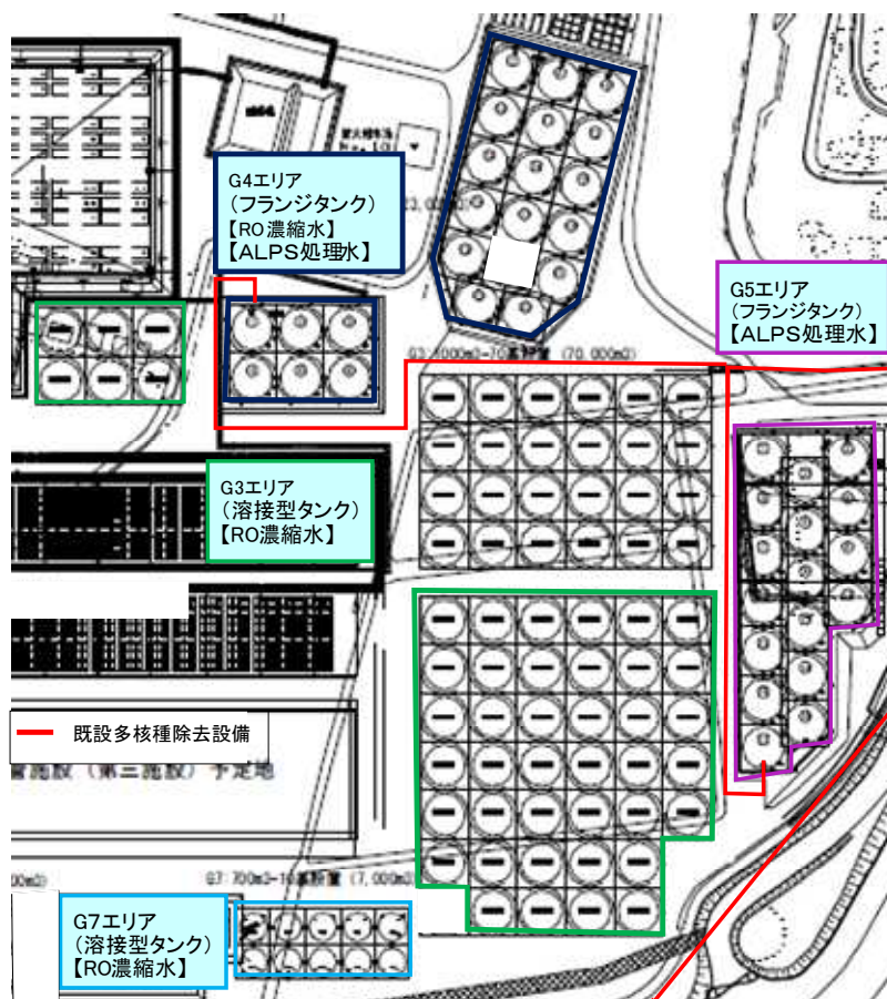
タンクエリア詳細図
