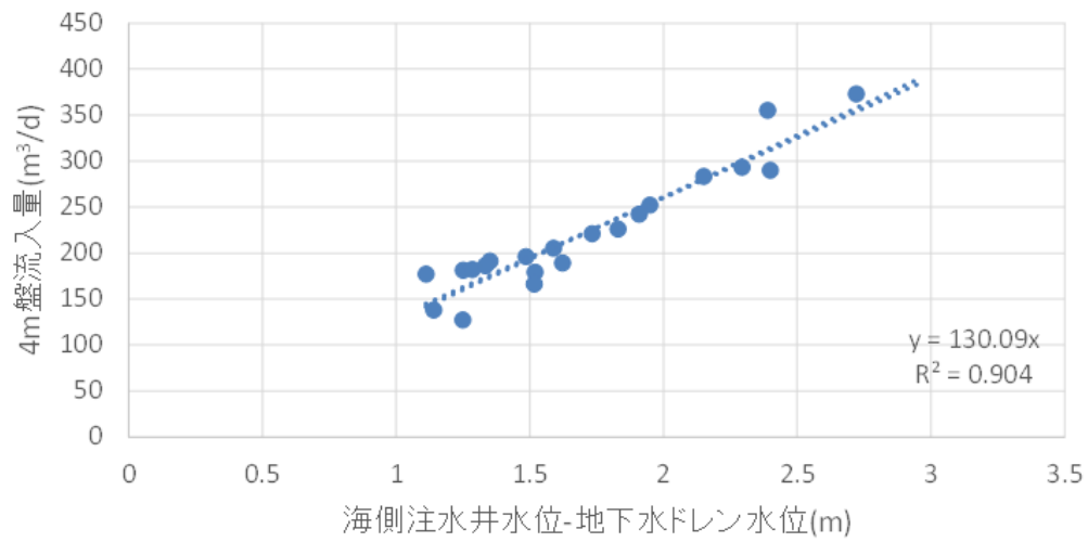
図－５ 海側注水井水位-地下水ドレン水位と4m盤流入量の関係 （期間：2016.7～2017.1）
