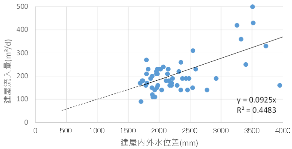
図－４ 建屋内外水位差と建屋流入量の関係（期間：2016.1～2017.1）
