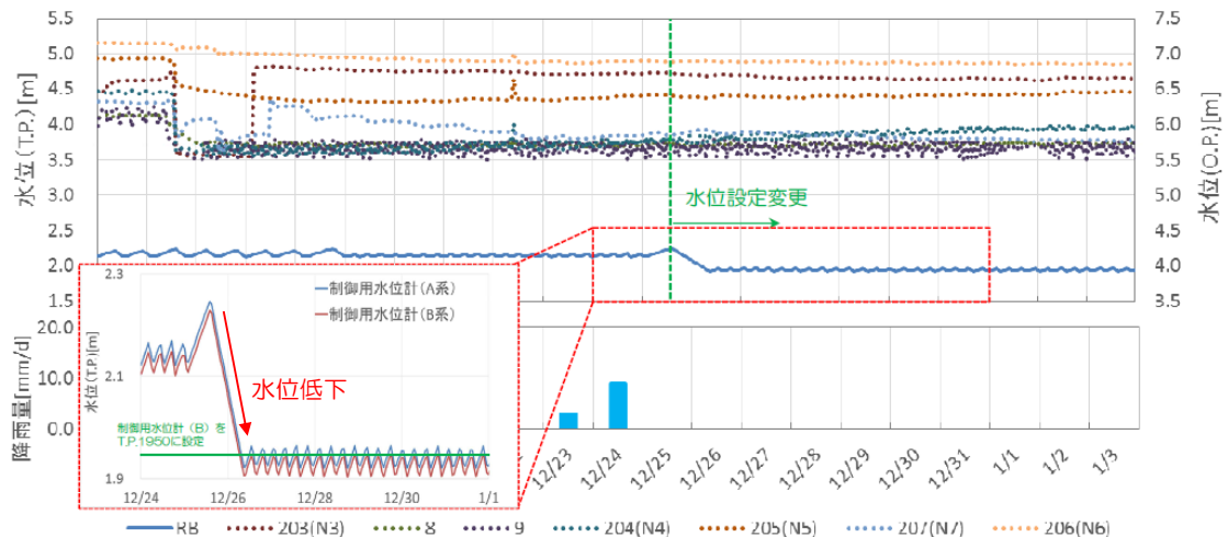
図-4 1号機原子炉建屋の建屋滞留水水位低下状況（実績）
