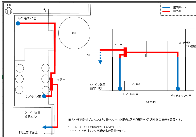
図－7 屋外排水ライン概略図
