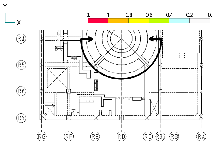
図-3.5.5 鉄筋ひずみの検定比 (シェル壁部)
