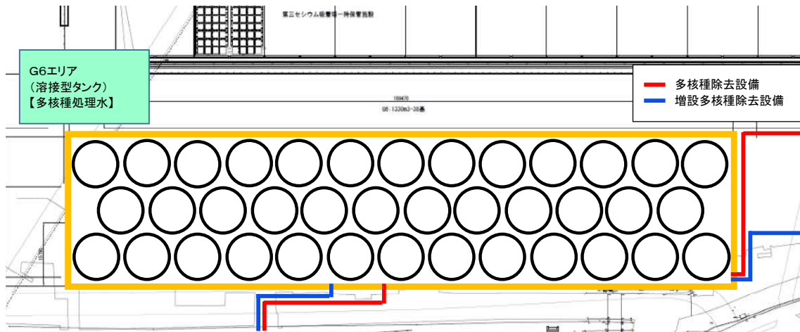
タンクエリア詳細図
