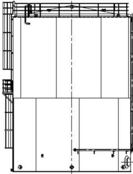
溶接型タンク概略図 (G6)
